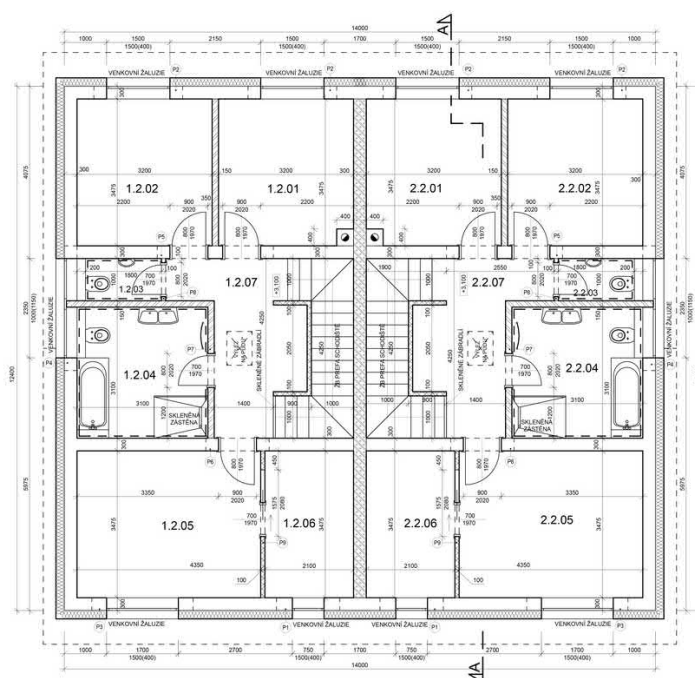
PŮDORYS 2.NP
