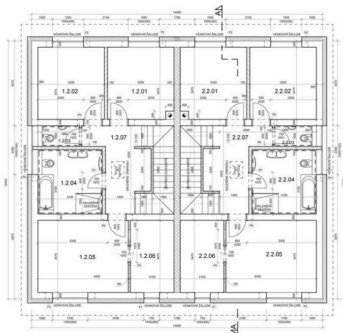
PŮDORYS 2.NP
