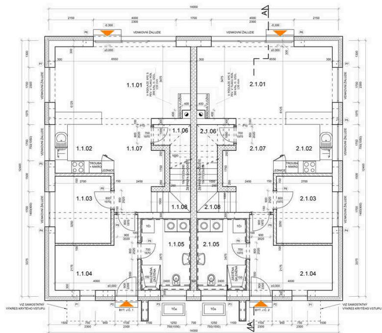
PŮDORYS 1.NP
